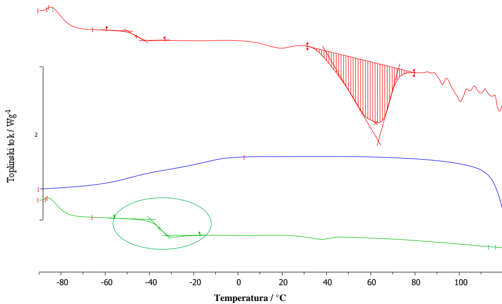
Slika 46. DSC krivulje uzorka PEO/5 % PEG-POSS/LiBOB (3. mjerenje)
