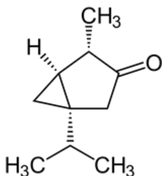
Slika 4. (+)- \alpha -tujon 27
