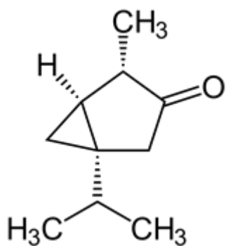
Slika 4. (+)- \alpha -tujon 27
