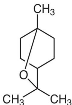
Slika 28. 1,8-Cineol 82
