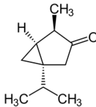
Slika 5. (-)- \beta -tujon 27
