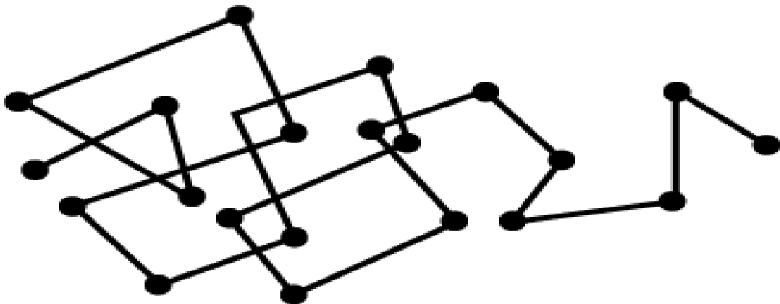
Slika 4. Brownovo gibanje 15
