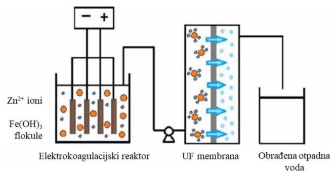
Slika 1.7. Shematski prikaz integracije elektrokoagulacije sa ultrafiltracijom. 14
