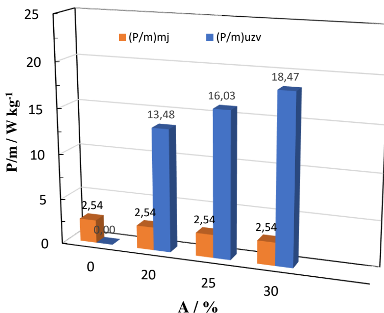
Slika 23. Snaga miješanja, (P/m)_{mj} i ultrazvučnog djelovanja, (P/m)_{uzv} , privedene sustavu pri različitim amplitudama ultrazvuka ( N_{JS} = 324 o. \text{min}^{-1} , T_z = 30^\circ\text{C} ).
