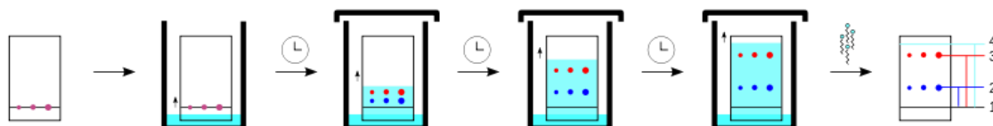
Slika 5. Tankoslojna kromatografija, razvoj kromatograma
