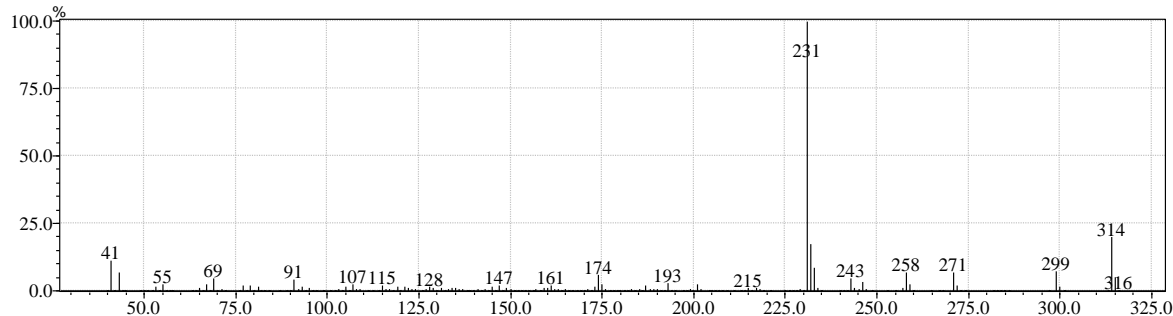
Slika 19. Karakterističan spektar masa za Δ-8-THC (m/z 231, 314, 258, 271)
