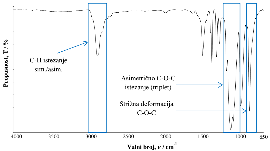
Slika 14. FT-IR spektar PEO
