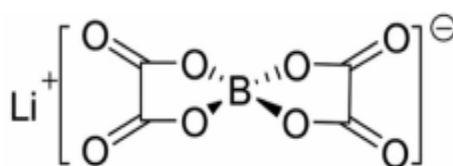
Slika 8. Struktura LiBOB 6
