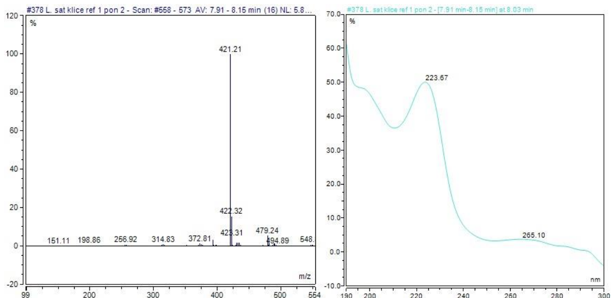
Slika 36. MS i UV spektar 4-metoksigliukobrasincina
