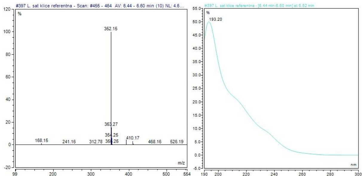
Slika 35. MS i UV spektar glutotropolina
