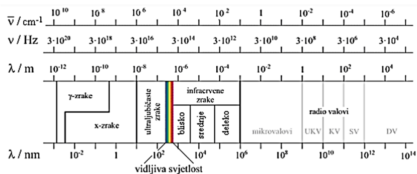
Slika 1.13. Elektromagnetski spektar. 29
