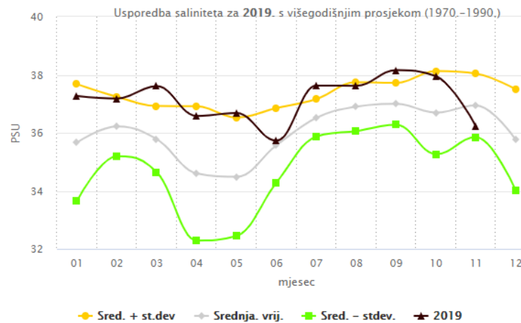
Slika 15. Godišnji hod saliniteta u površinskom sloju postaje OC06 (Kaštelanski zaljev) [25]
