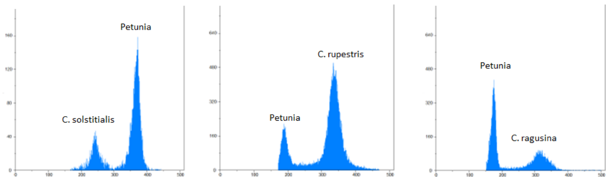
Slika 11. Histogramski prikaz veličine genoma kod proučavanih vrsta roda Centaurea (28)
