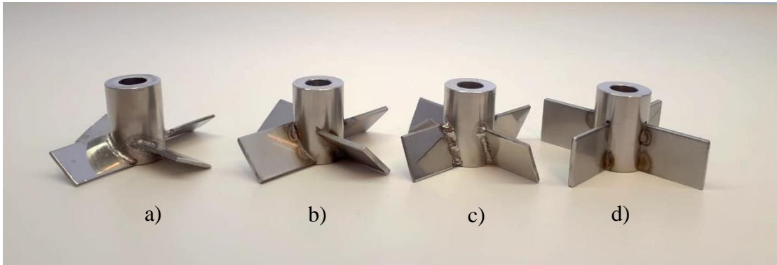
Slika 14. Turbinska miješala različitih nagiba lopatica: a) 30^\circ , b) 45^\circ , c) 70^\circ , d) 90^\circ
