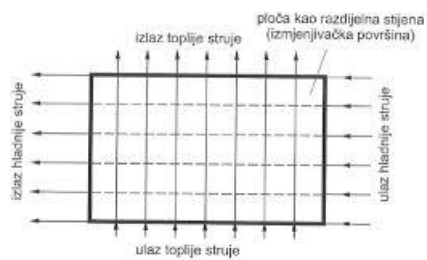
Slika 8. Križni tip rekuperatora 6
