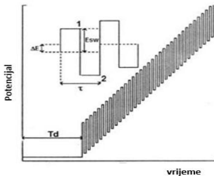
Slika 12. Pravokutni izmjenični signal pobude pravokutnovalne voltetrije [14].
