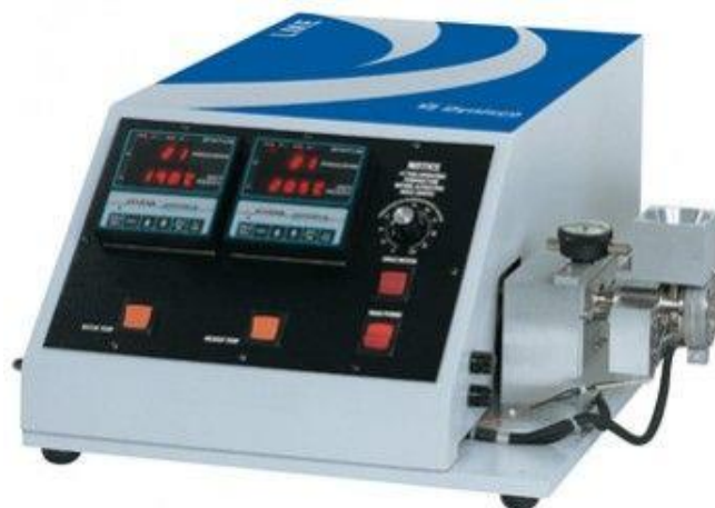
Slika 12. Laboratorijski jednupužni ekstruder Dynisco (Qualitest, SAD)
