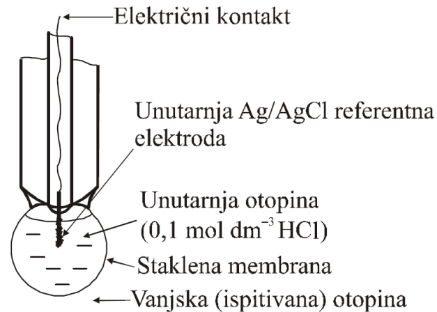
Slika 8. Staklena elektroda 1
