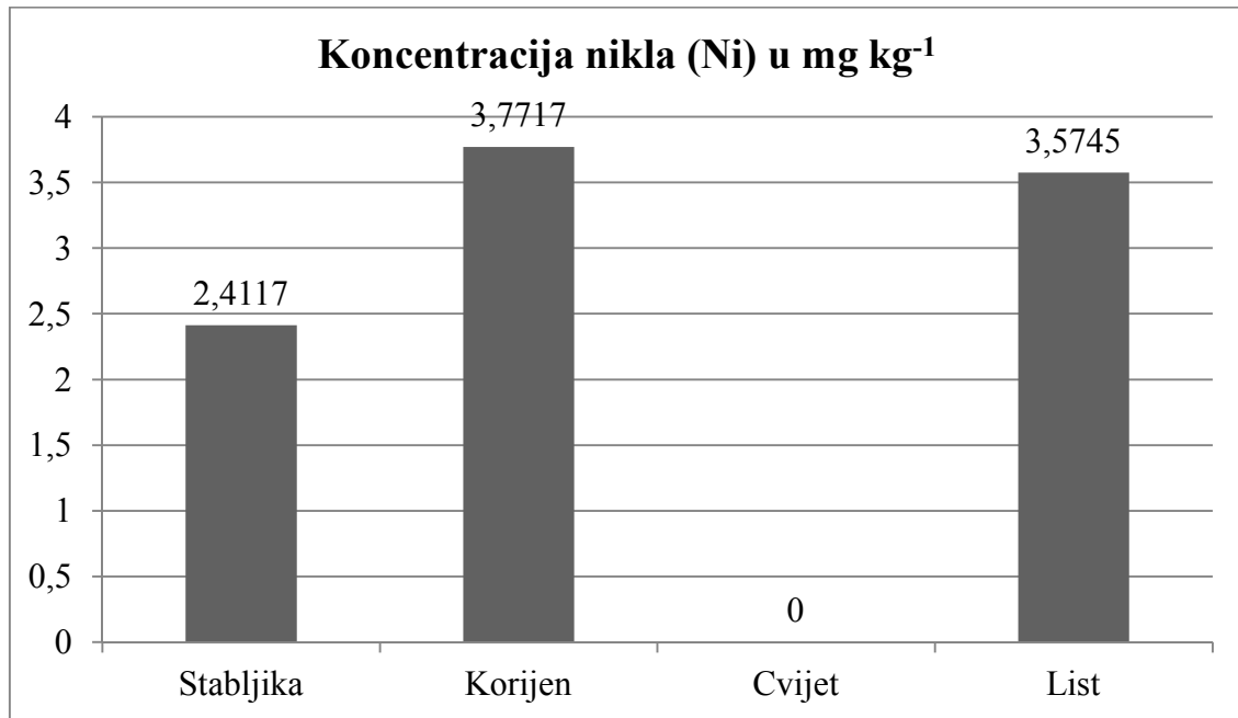
Slika 20. Koncentracija nikla u ispitivanom uzorku
