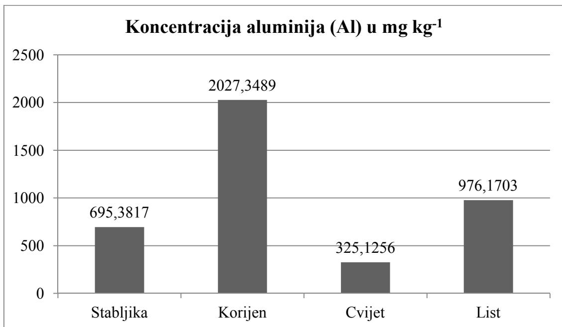
Slika 21. Koncentracija aluminija u ispitivanim uzorcima
