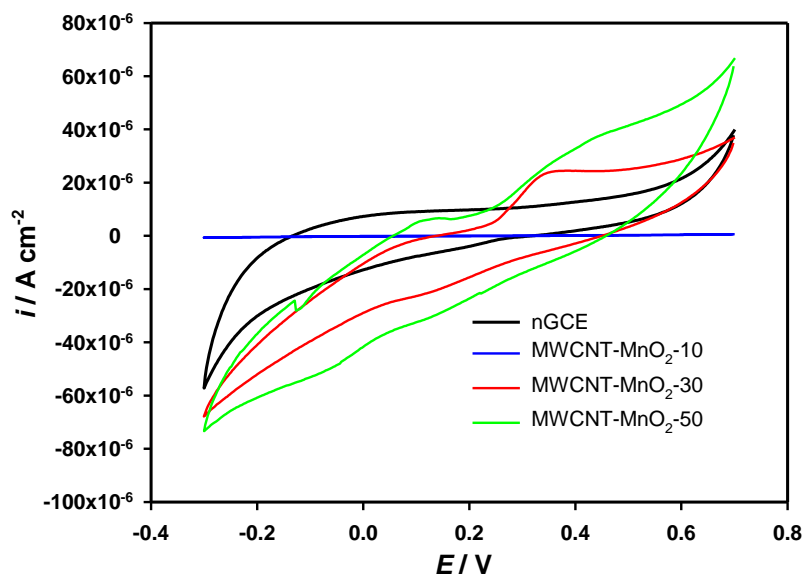
Slika 25. CV snimljeni pri pH 9 za različite količine kompozita s MWCNT- MnO_2 .
