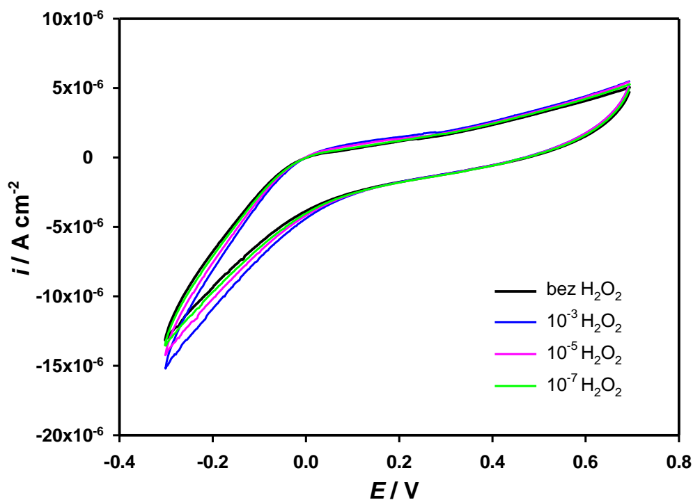
Slika 20. Utjecaj dodatka H_2O_2 na CV u acetatnom puferu (pH 5). GCE-MWCNT-30
