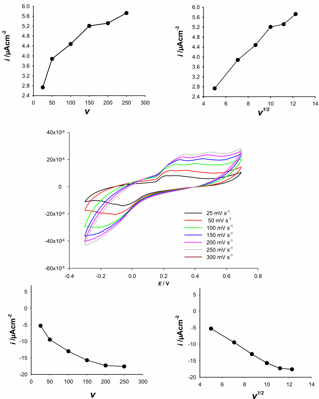
Slika 35. Utjecaj posmika na CV elektrode MWCNT-AgCuS-30 u otopini puferiranoj amonijakalnim puferom (pH 9), pri konc. H_2O_2 1 \times 10^{-3} \text{ mol dm}^{-3} . Ovisnost anodnih i katodnih struja pika o posmiku i njegovom korijenu.
