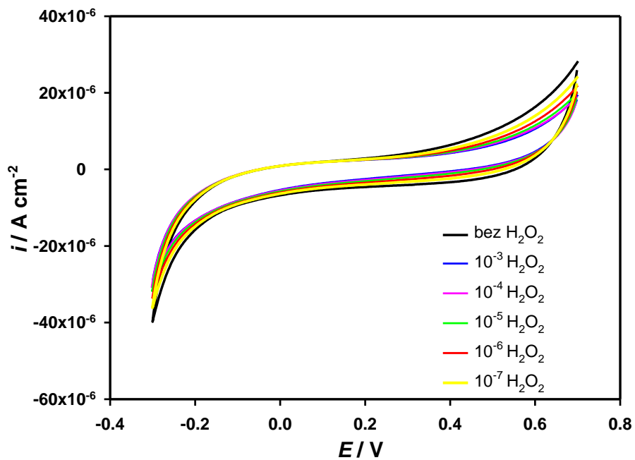
Slika 15. Utjecaj dodatka H_2O_2 na CV u fosfatnom puferu (pH 7). GCE elektroda
