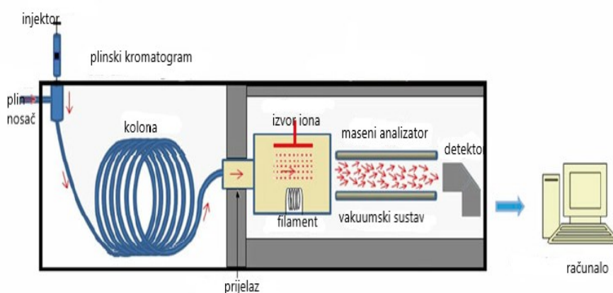
Slika 14. Vezani sustav GC-MS 12
