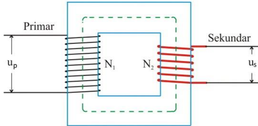
Slika 2.10. Transformator.
