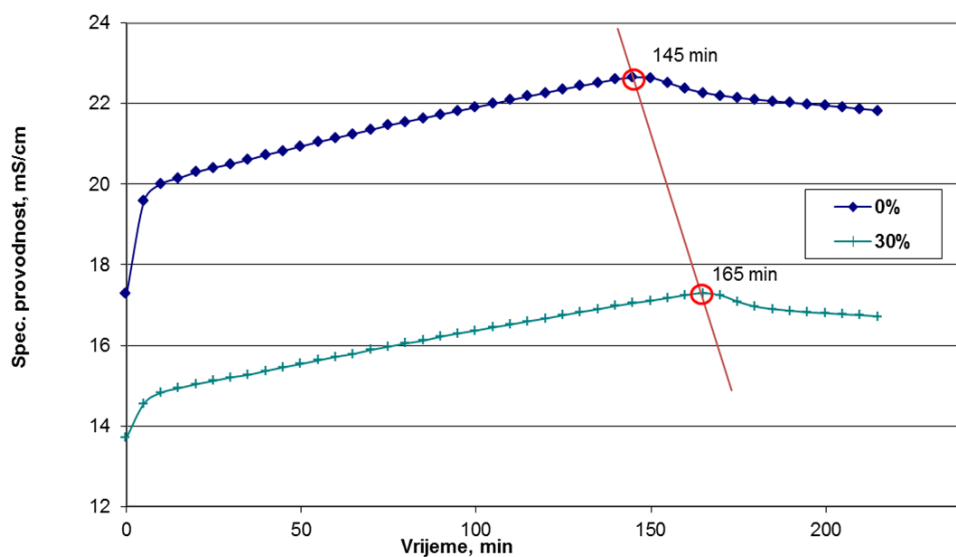
Slika 19: Ovisnost vremena pojave maksimuma specifične provodnosti cementnih pasti bez dodatka otpadne građevinske opeke i sa 30% dodatka.
