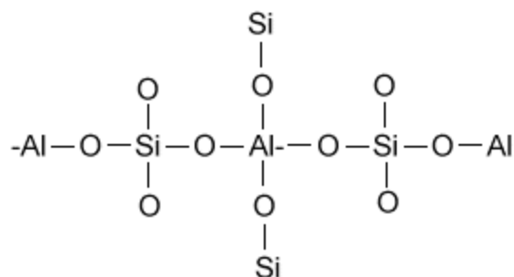
Slika 2. Struktura zeolita 9
