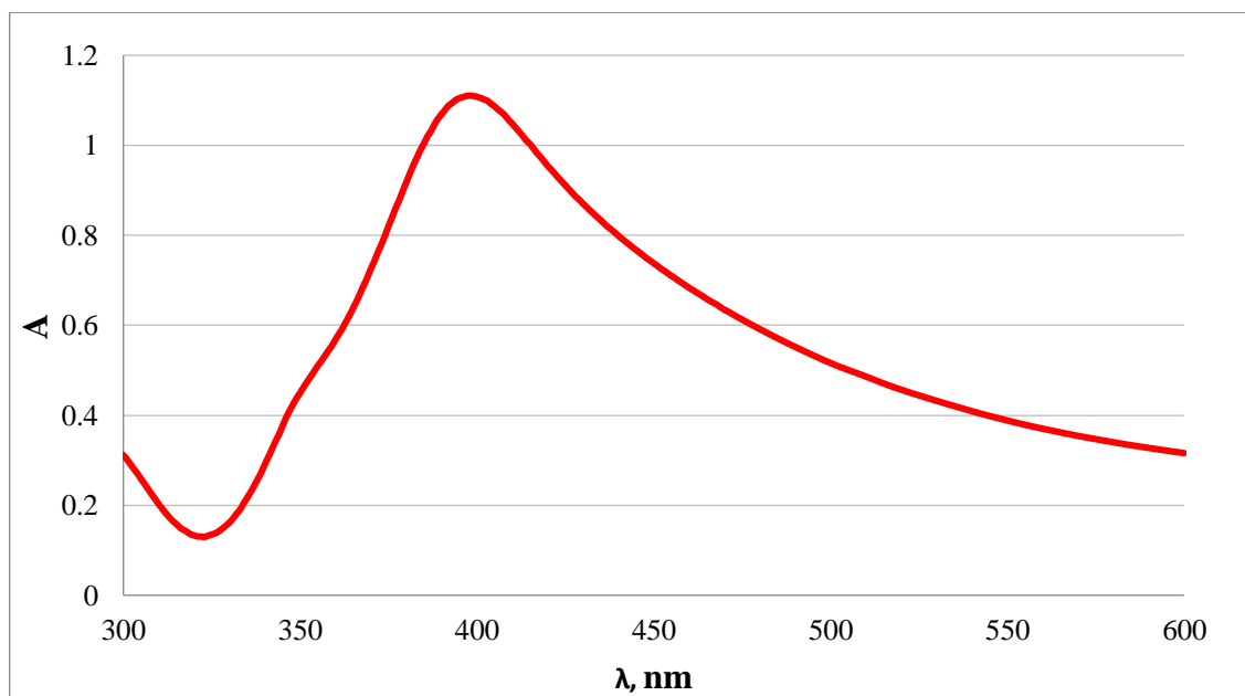
Slika 16. Apsorpcijski spektar koloidnog srebra dobivenog pomoću 0,008% natrijevog borohidrida
