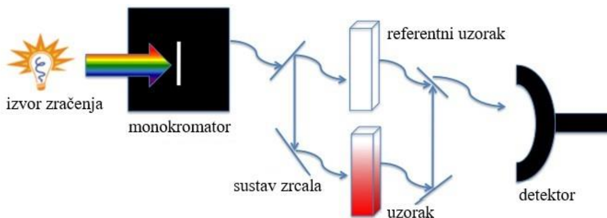
Slika 18. Dvozračni spektrofotometar 32
