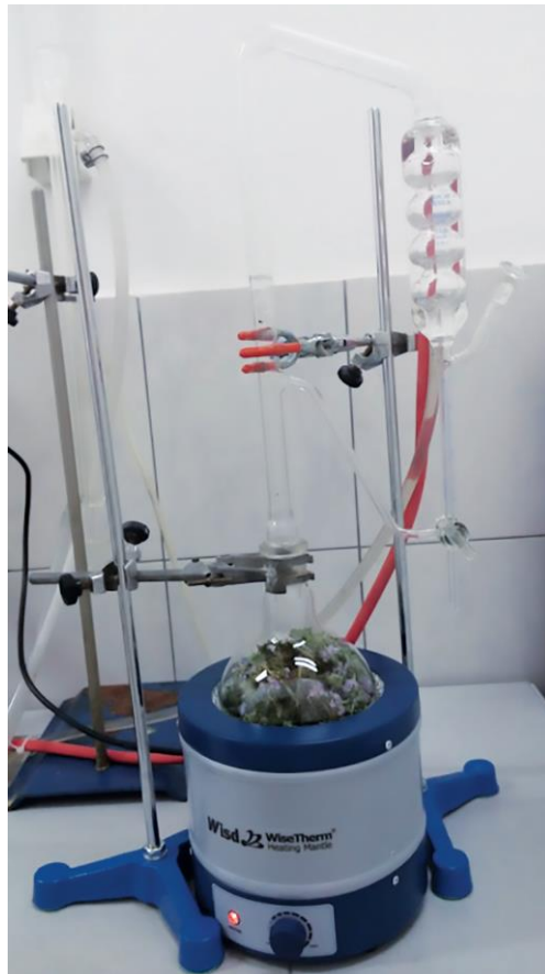
Slika 3.2. Aparatura po Clevengeru
