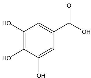
galna kiselina
