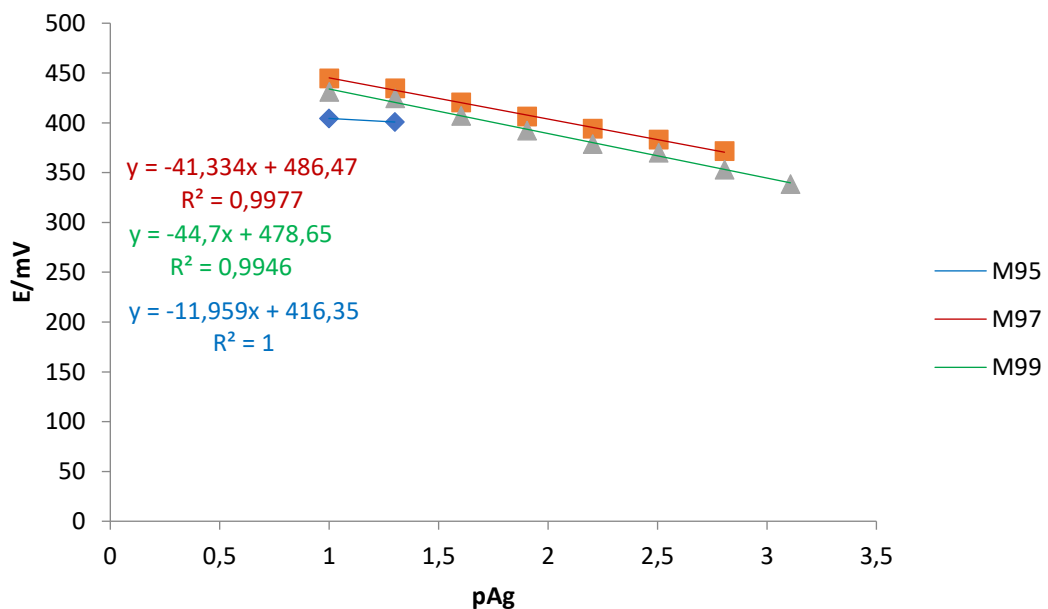
Slika 14. Prikaz testiranja odziva elektrode na Ag +
