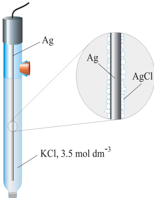
Slika 4. Elektroda Ag/AgCl 3
