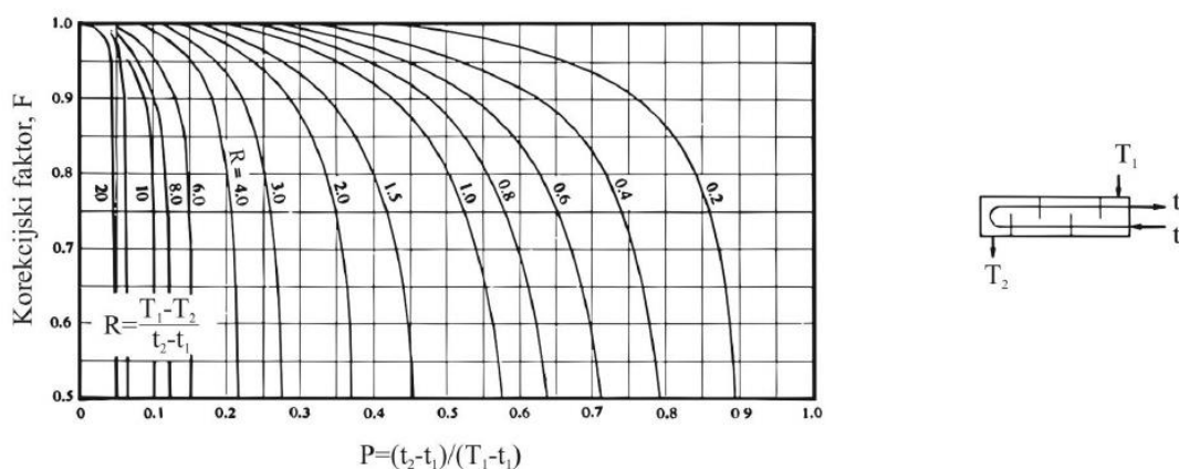
Slika 12. Dijagram ovisnosti 6 F = f(P, R) za protusmjerni izmjenjivač tipa 1-2
