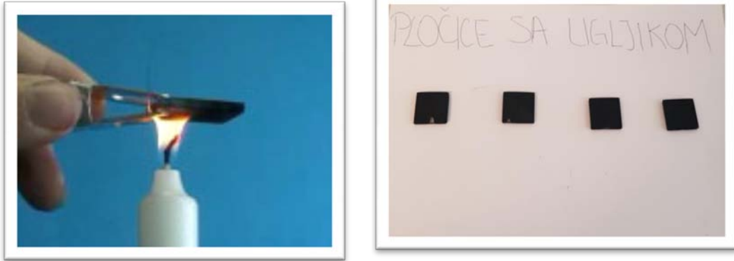
Slika 15. Nanošenje ugljičnog sloja
