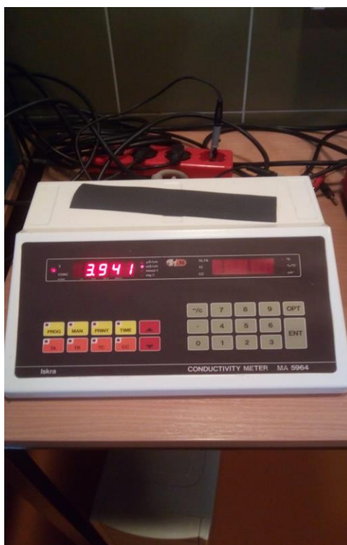
Slika 5. Aparatura korištena za određivanje specifične provodnosti: a) osobno računalo b) mjerna posuda u termostatiranoj vodenoj kupelji c) konduktometar MA 5964 – ISKRA
