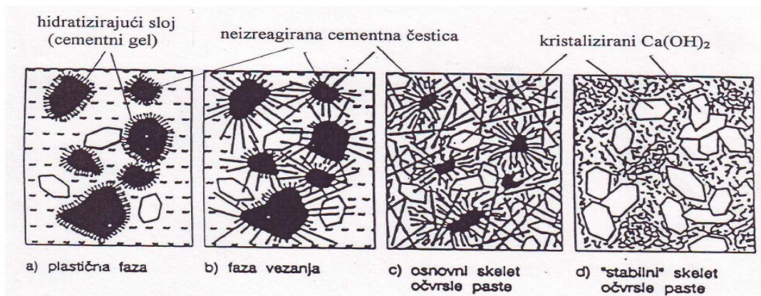
Slika 2. Shematski prikaz stvaranja strukture očvrsl cementne paste 4
