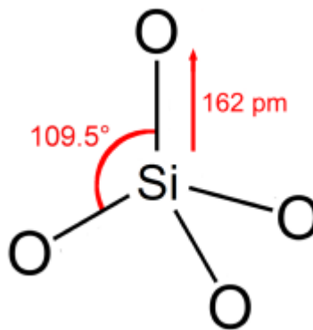
Slika 1. Tetraedar silicija
