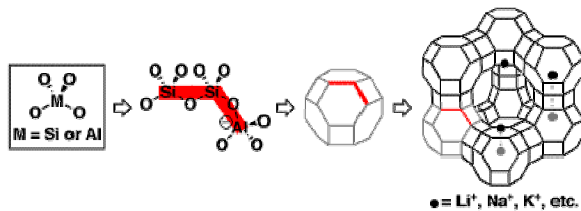
Slika 1.8. Struktura zeolita 15
