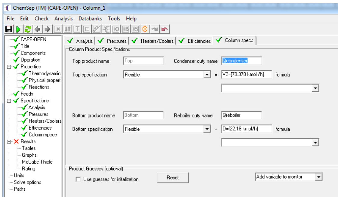
Slika 2.10. Specifikacija uvjeta razdvajanja destilacije kolone u ChemSep-u.
