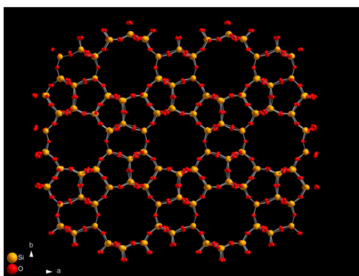
Slika 8. Zeolit ZSM-5 20
