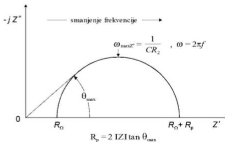
Slika 15. Nyquistov prikaz
