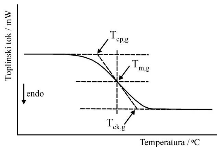
Slika 8. Određivanje staklišta
