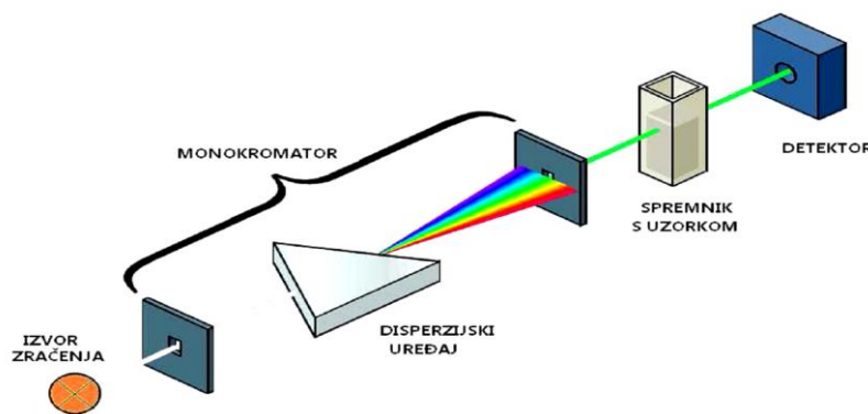
Slika 1.31. Shematski prikaz spektrofotometra.
