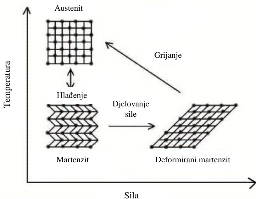
Slika 2. Ciklus promjena strukture za SMA legure (5)
