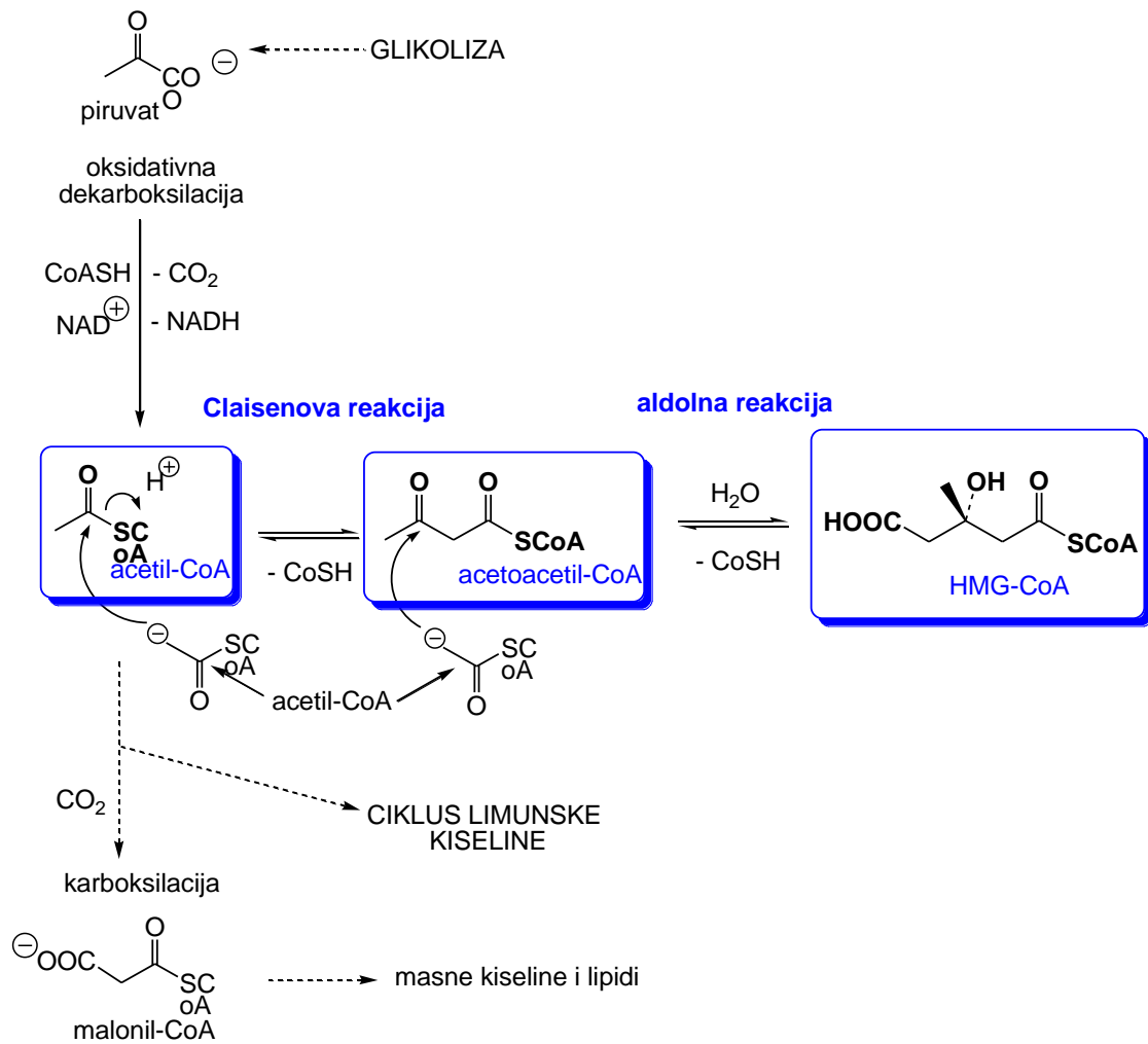
Slika 12. Biosinteza β-hidroksi-β-metilglutaril-CoA (HMG-CoA)
