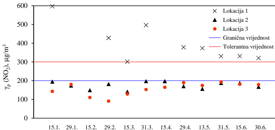
Slika 4.2. Usporedba graničnih i tolerantnih vrijednosti emisija s izmjerenim vrijednostima emisija koncentracija NO 2 za tri lokacije za šestomjesečni mjerni period.
