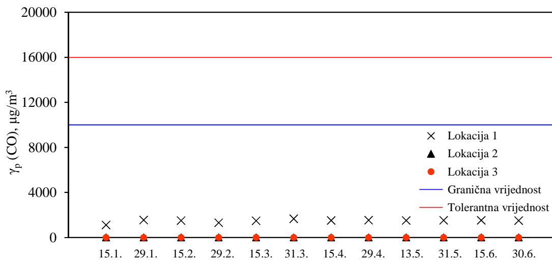
Slika 4.3. Usporedba graničnih i tolerantnih vrijednosti emisija s izmjerenim vrijednostima emisija koncentracija CO za tri lokacije za šestomjesečni mjerni period.
