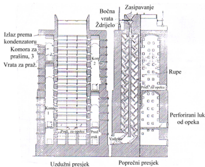
Slika 1.5. Scottova presipna peć 8
