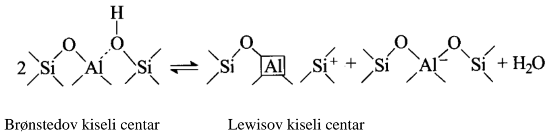
Slika 8. Brønstedovi i Lewisovi kiselinski centri u zeolitima 3
