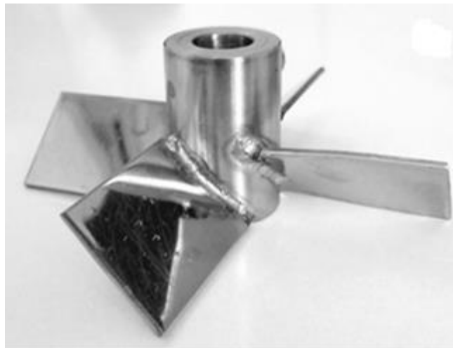
Slika 15. PBT miješalo
