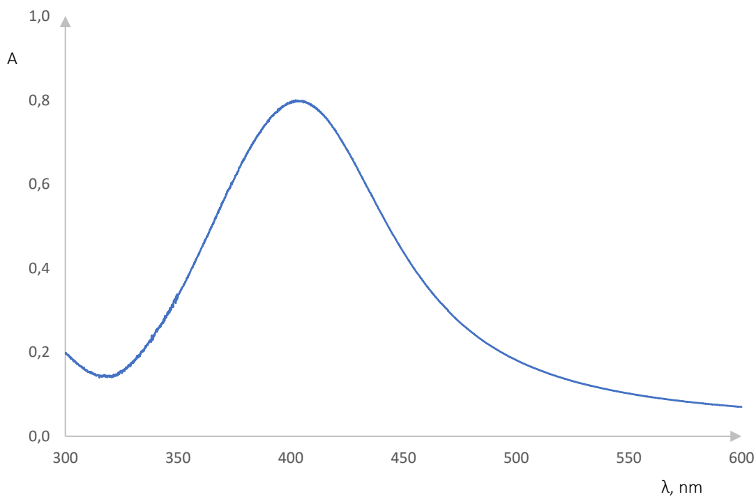
Slika 38. Apsorpcijski spektar pri koncentraciji AgNO 3 0,0005 mol/dm 3
