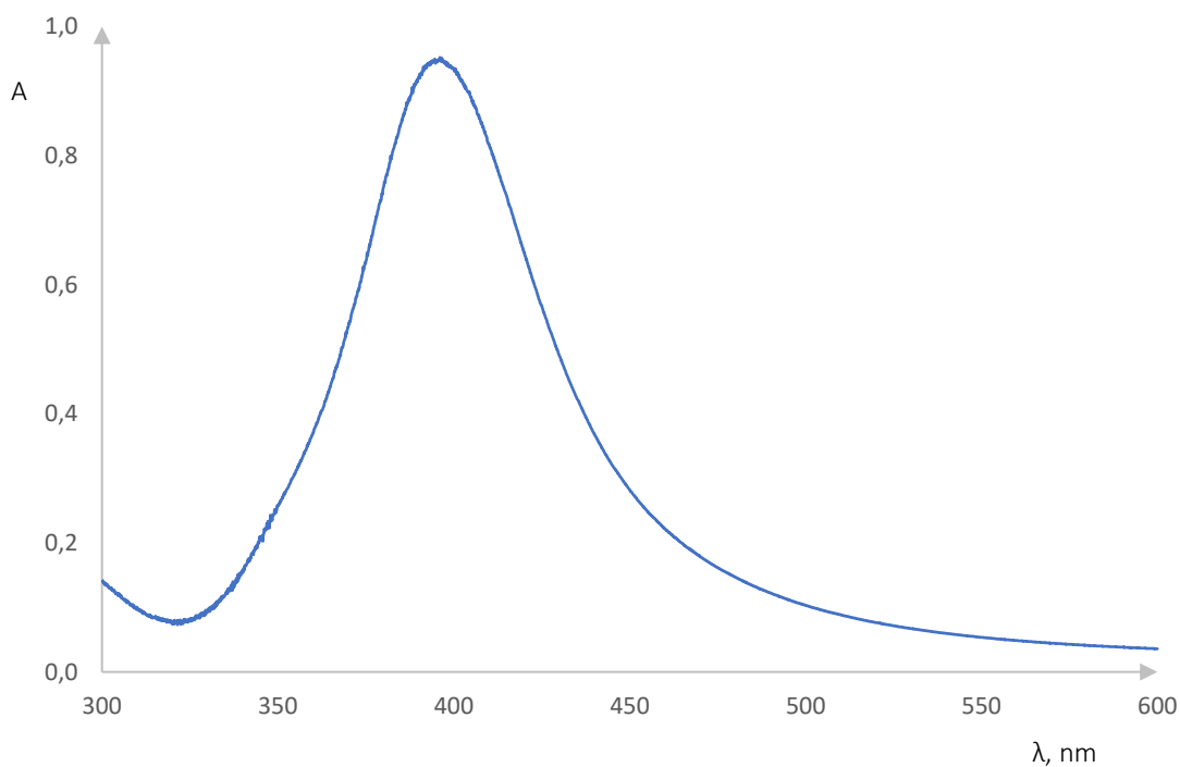
Slika 37. Apsorpcijski spektar pri koncentraciji AgNO 3 0,0020 mol/dm 3
