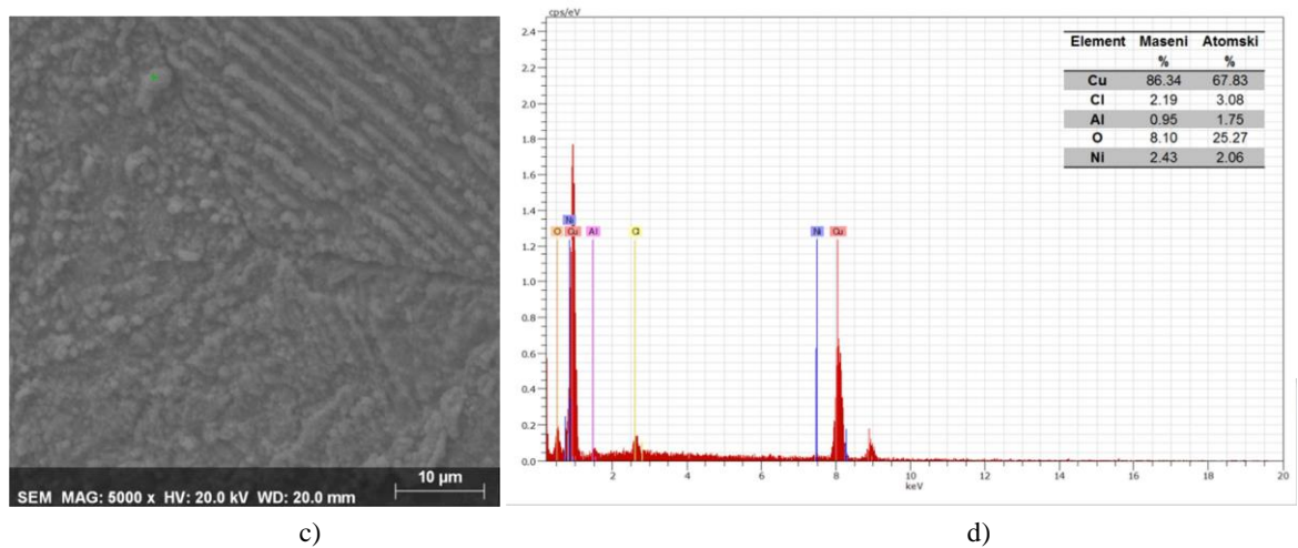
Slika 34. SEM snimka površine uzorka CuAlNi legure nakon potenciodinamičkog polarizacijskog mjerenja u 1.5 % NaCl otopini i pripadajuća EDS analiza
