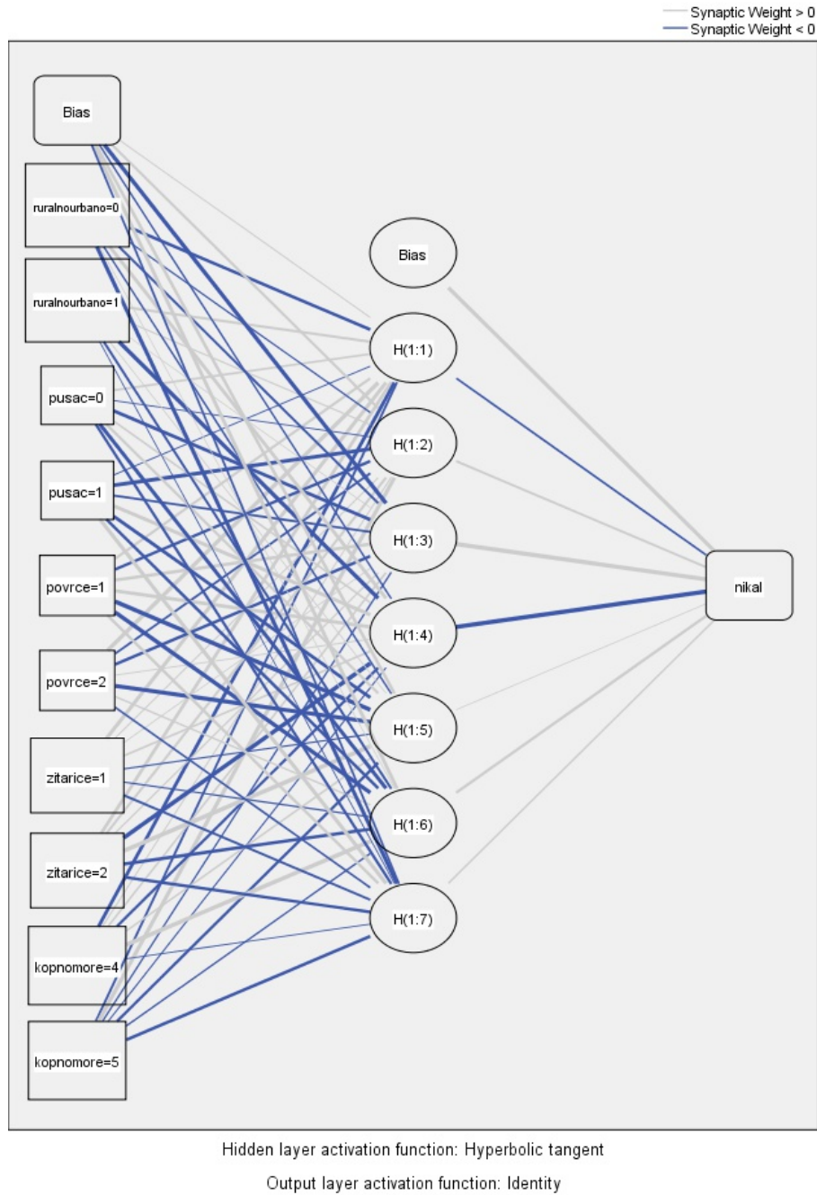
Slika 5.37. Algoritam umjetne neuronske mreže za nikal.
