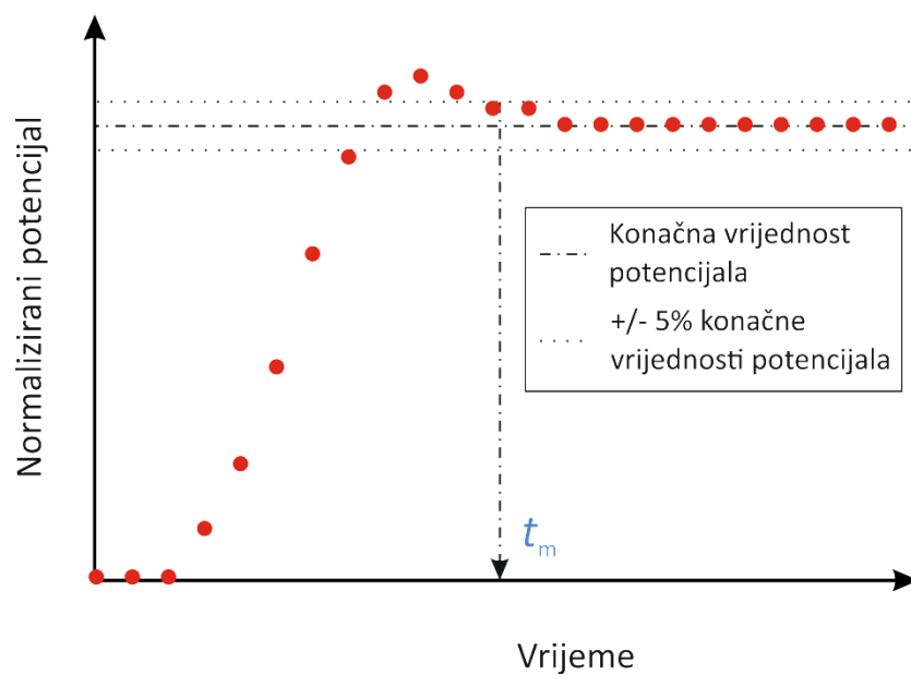
Slika 31. Određivanje vremena homogenizacije iz promjene potencijala otopine.
