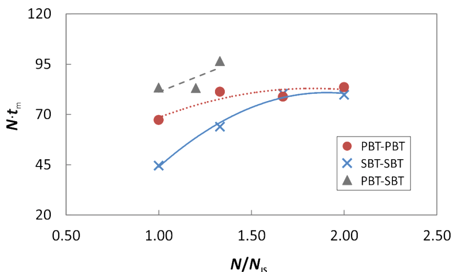
Slika 44. Vrijeme homogenizacije svih ispitivanih konfiguracija miješala u ovisnosti o brzini vrtnje miješala.
