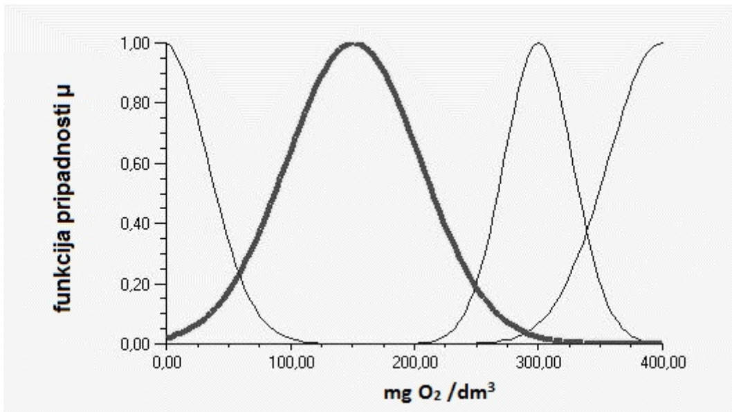
Slika 51. Stupanj pripadnosti iz podataka za BPK 5 s jezičnim terminom „korektan“
