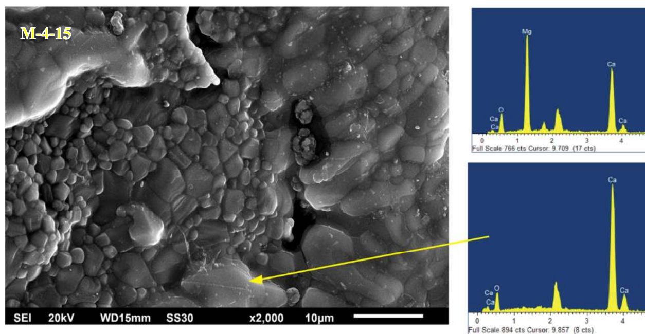
Slika 4.51. SEM/EDS snimka uzorka magnezijeva oksida (80% tno taloženje) dobivenog iz morske vode bez dodatka \text{TiO}_2 uz pripadajuću elementarnu analizu karakterističnog područja ( t = 1500 °C uz vrijeme izoternog sinteriranja \tau = 4 h).
