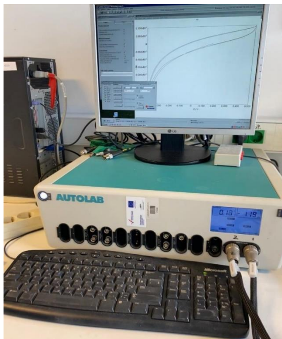
Slika 26 Uređaj za voltometrijska mjerenja
