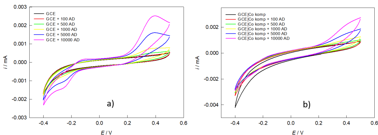
Slika 27 Ciklički voltamogrami snimljeni na GCE (a) i GCE|Cokomp (b) s različitom koncentracijom adrenalina dodanog u osnovni elektrolit. ( v = 25 \text{ mV s}^{-1} )
